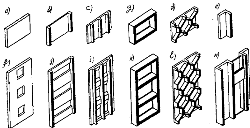
Hình VIII.7- Hệ panen tường chịu lực phía ngoài a,f- panen đặc ; b,c,z,i- panen có gờ ; g,k- panen có mặt cắt dạng cổ kim ; d,l- panen khung dạng lưới ; e,m- panen không gian.
