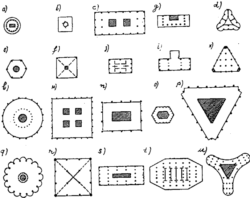
Hình IV.15. Nhà khung có lõi cứng
