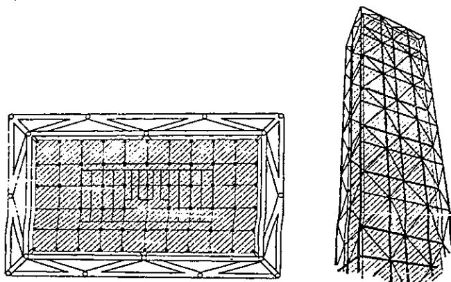
Hình IV.20- Tháp do S.Venxon đề xuất
