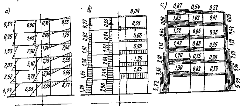
Hình VI.43 Biểu đồ nội lực
