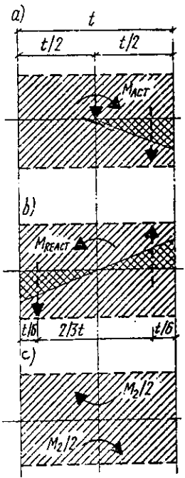
Hình VI.18 1- Tầng 2 (a,b,c)
