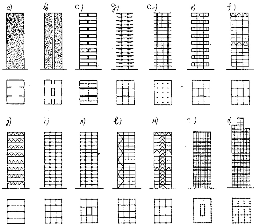
Hình II.1. Những sơ đồ kết cấu của nhà cao tầng
