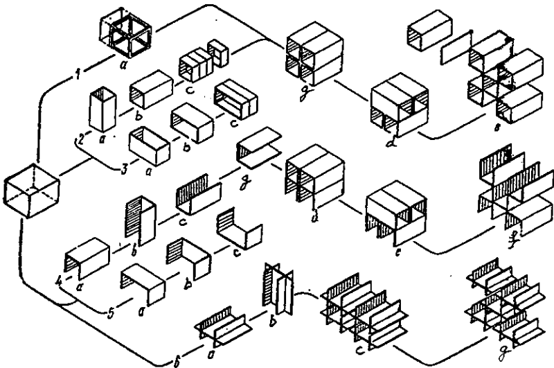
Hình VIII.10. Các bloc hình khối môđun chính
