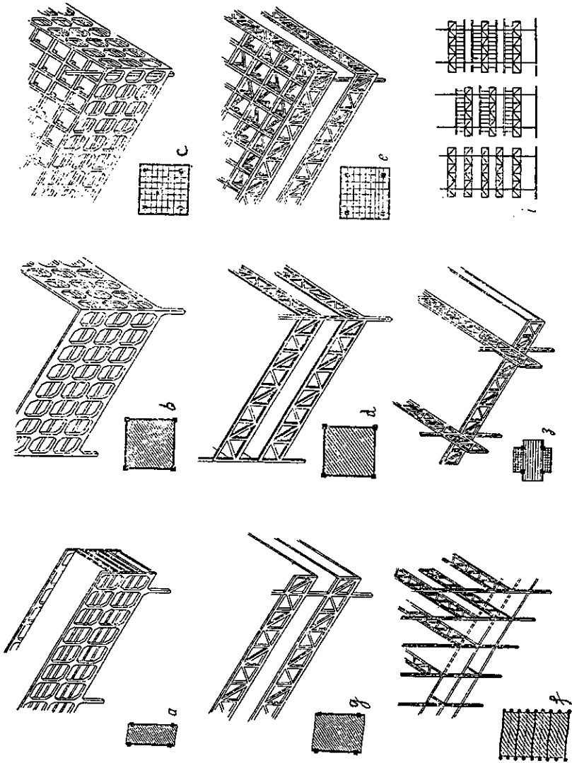
Hình IX.1 Hệ có dầm cao
