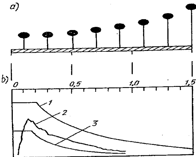
Hình I.17 1- Phổ ứng xử không tính tới độ tắt dần; 2- Phổ ứng xử ghi được; 3- Phổ ứng xử khi kể đến độ tắt dần.
