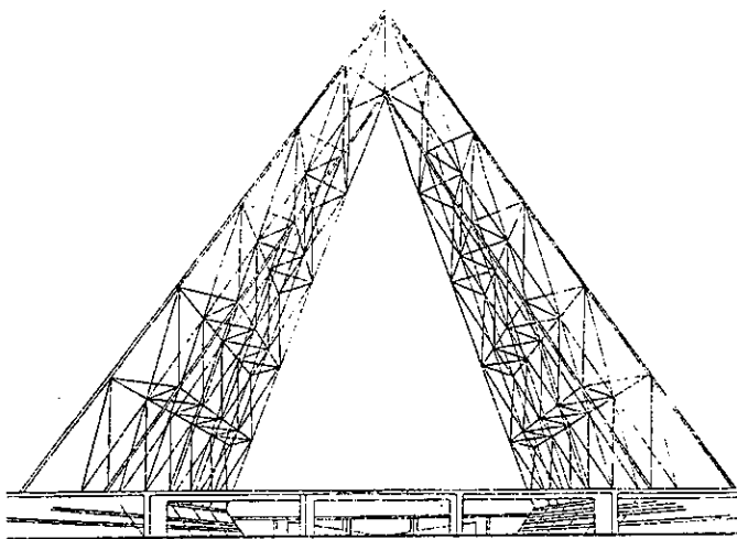
Hình IX.21- Khung không gian chữ A do Chighecan đề xuất
