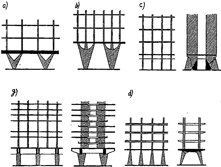
Hình III.13 Hệ thống kết cấu đỡ ở tầng dưới cùng
