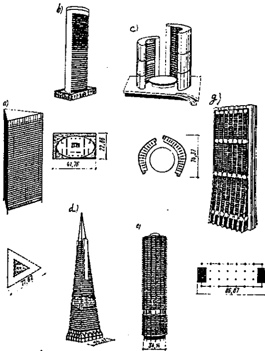
Hình V.1- Hình dạng hợp lý của ngôi nhà
