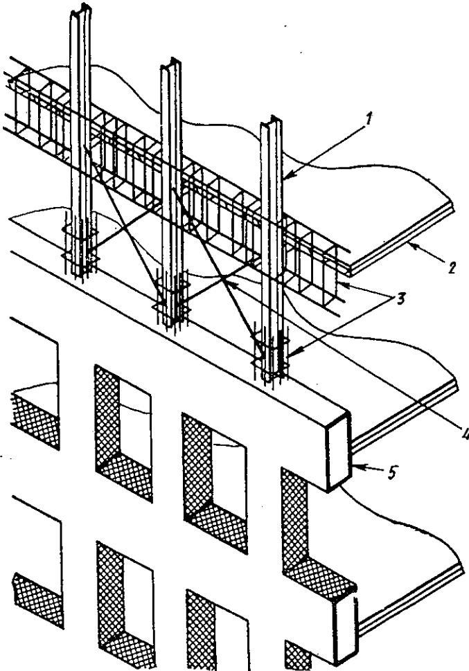
Hình IV.31. Sơ đồ nhà có kết cấu hộp liên hợp
