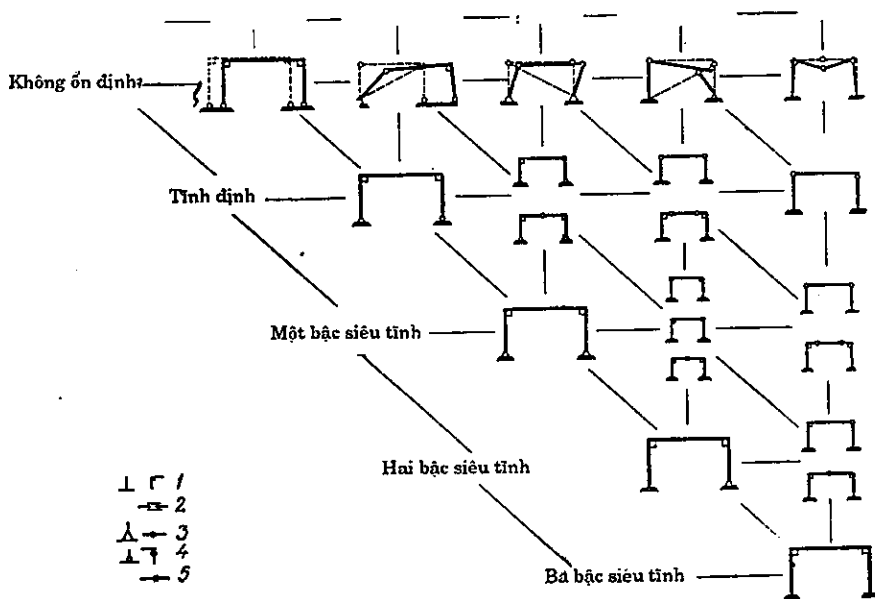
Hình VIII.2- Các dạng chính của khung chữ \Pi
