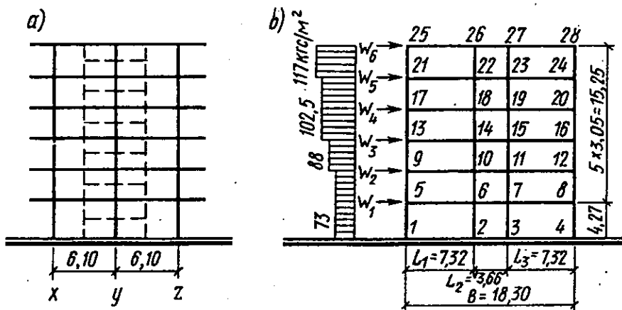
Hình VI.37 a - Mặt cắt ; b - Sơ đồ khung trục y
