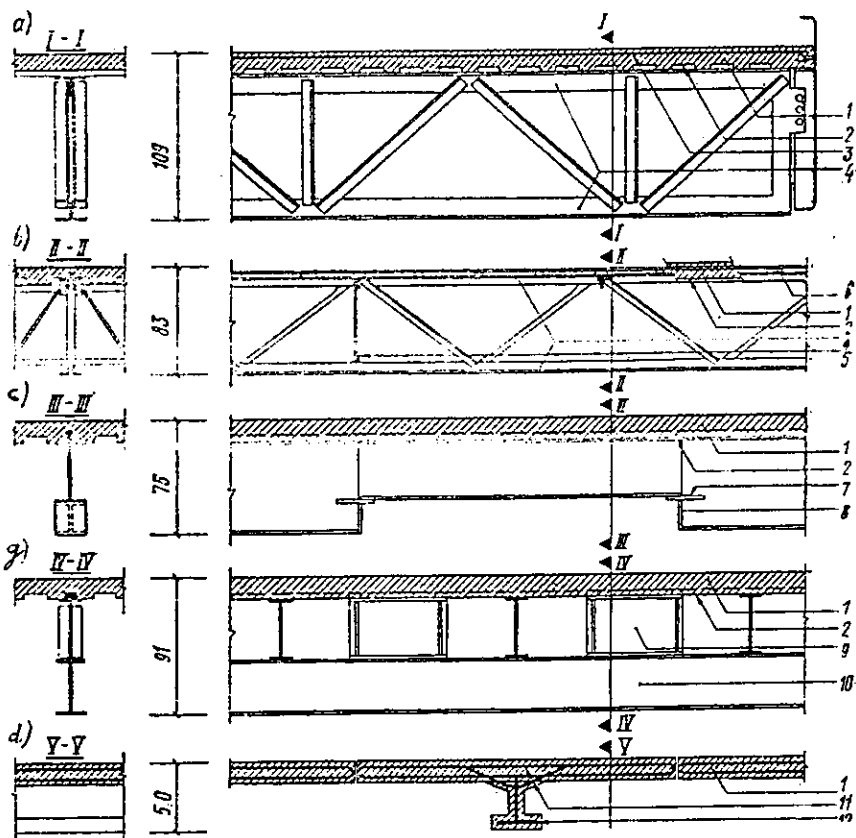
Hình VII.5. Hệ sàn liên hợp
