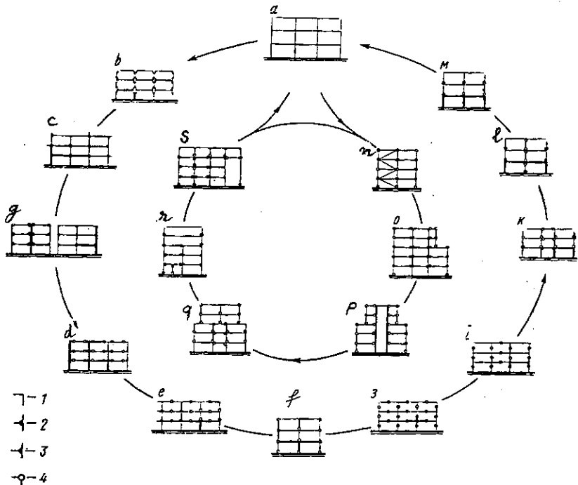
Hình VIII.3- Hệ cấu kiện môđun cho nhà khung
