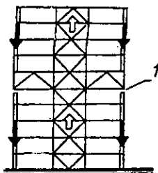
Hình 1.43 1- Khe nhiệt
