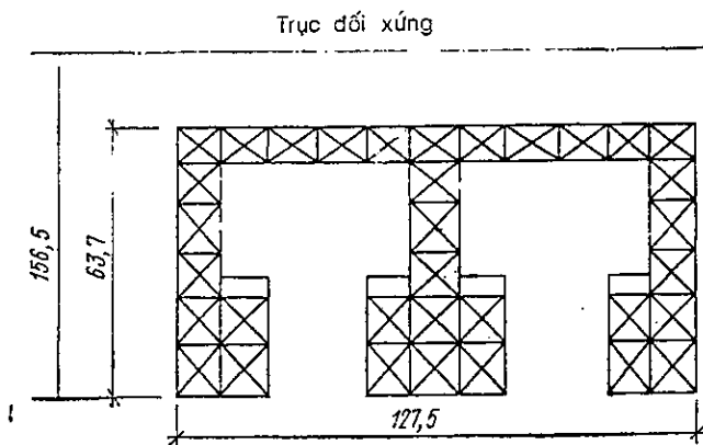
Hình IX.19- Mặt bằng ngôi nhà VAB
