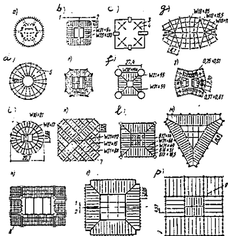
Hình VII.3. Những kết cấu sàn thông dụng
