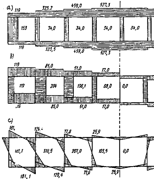
Hình VI.63 : Biểu đồ nội lực
