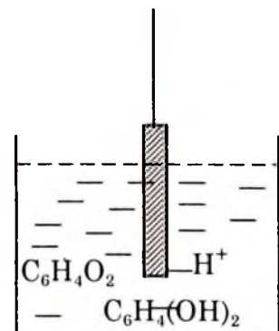
Hình 8.8. Cấu tạo của điện cực quinhydron
