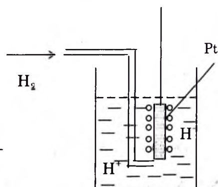
Hình 8.5. Cấu tạo của điện cực khí hydro
