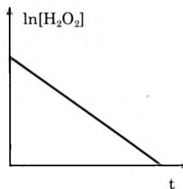
Hình 4.6. Đồ thị phản ứng bậc 1 sự phân huỷ H_2O_2
