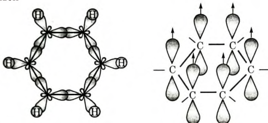
Hình 2.12. Các orbital p thuần và sự hình thành liên kết \pi không định cư trong phân tử benzen
