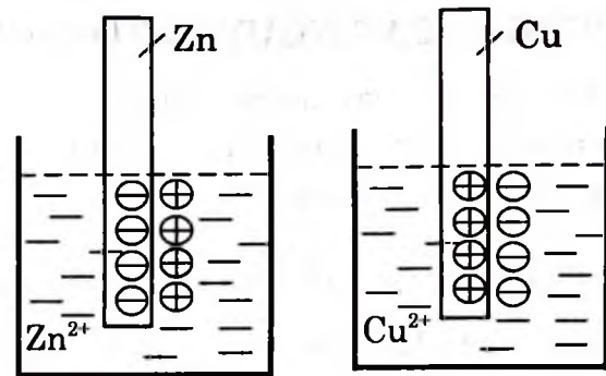
Hình 8.2. Sự hình thành lớp điện kép trên điện cực
