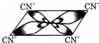
Hình 2.16. Các orbital lai hoá d s 2 của Ni 2+ và sự tạo thành ion phức [Ni(CN) 4 ] 2-
